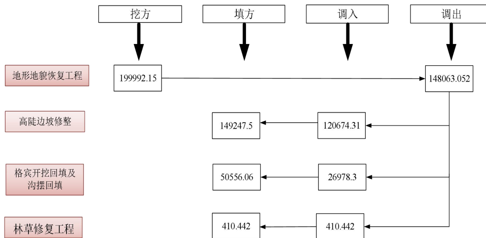
图 2-4 土石方平衡框图 (单位: m³)
